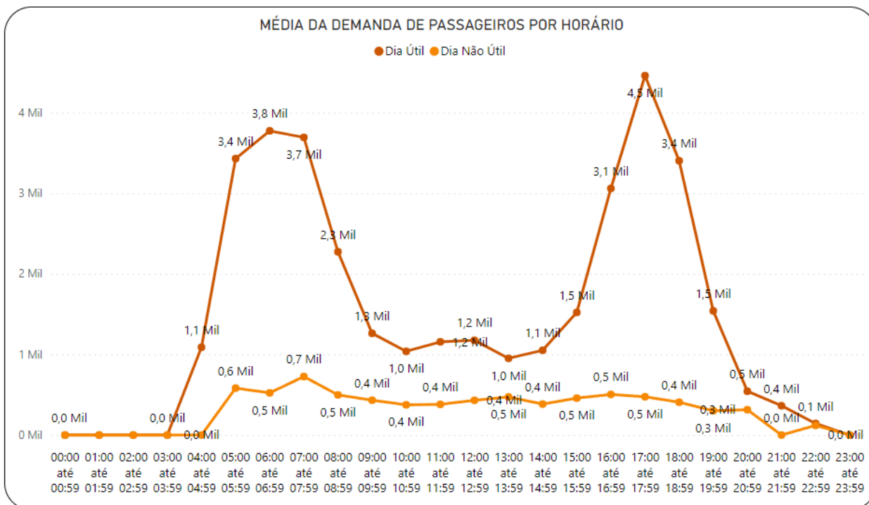
Gráfico 3-77 Demanda Horária – Gramacho – ago/2023
