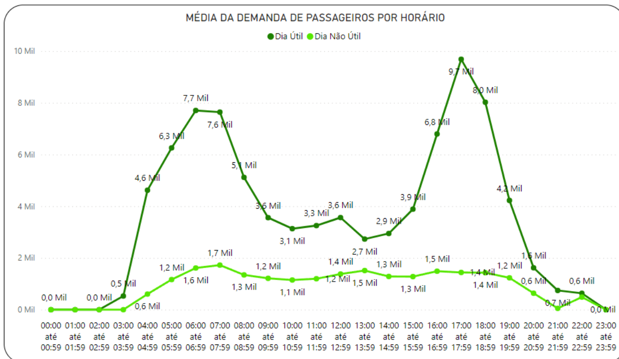
Gráfico 3-79 Demanda Horária – Santa Cruz – ago/2023
