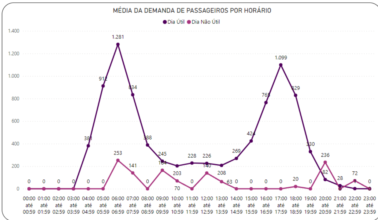
Gráfico 3-76 Demanda Horária – Belford Roxo – ago/2023
