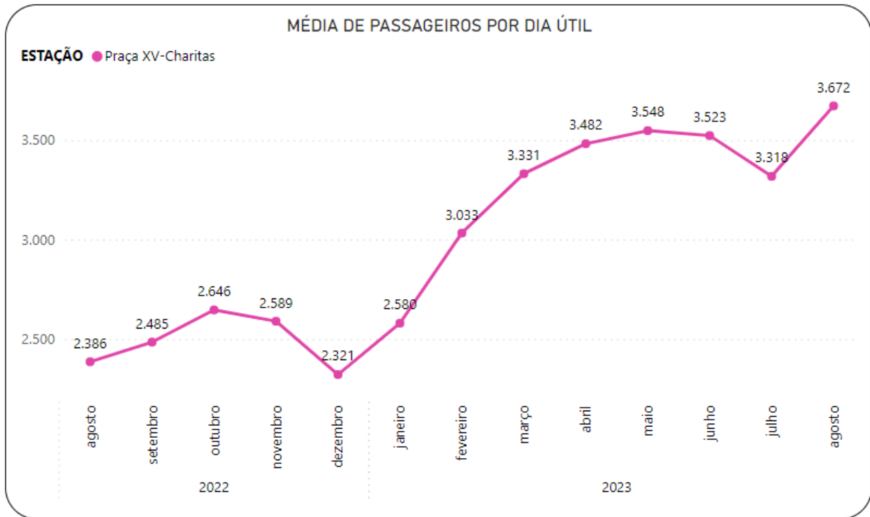
Gráfico 3-10 CCR Barcas – Média de Passageiros Transportados nos Dias Úteis s – Praça XV - Charitas
